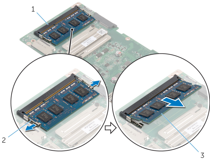
2 תפסי הידוק (2)
